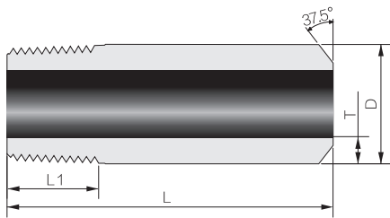
单头短节
