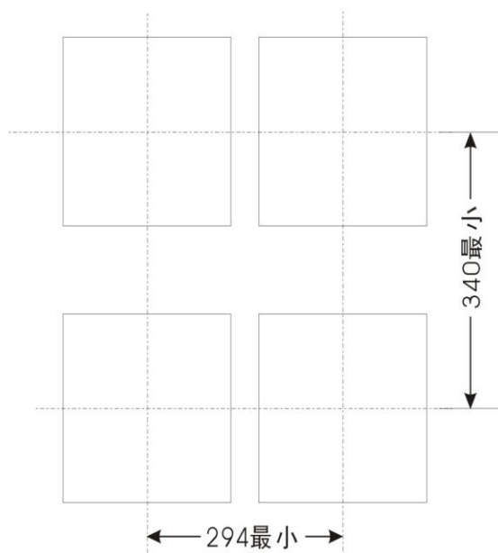
集装表开孔尺寸
