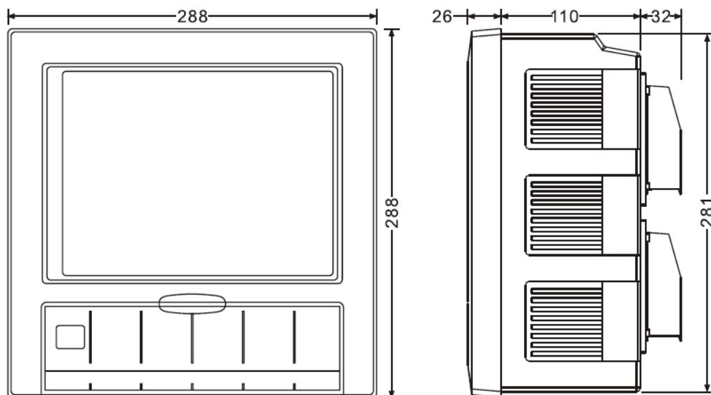
仪表外形尺寸
