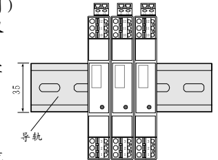
垂直安装示意图
