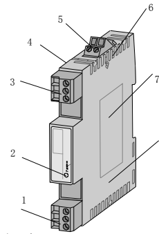
产品结构立体图
